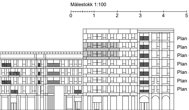
Fasade, Vest
