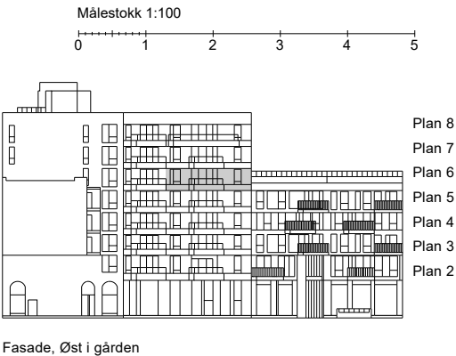
Fasade, Øst i gården
